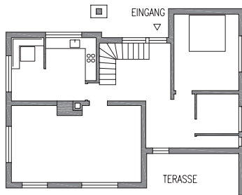
ERDGESCHOSS BESTAND
